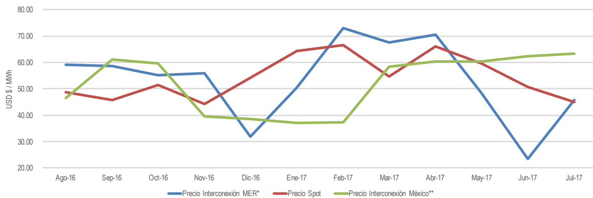
Promedio Precio MER, Interconexión México y Precio Spot
