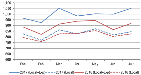
Resumen de Consumo de Energía (GWh)
