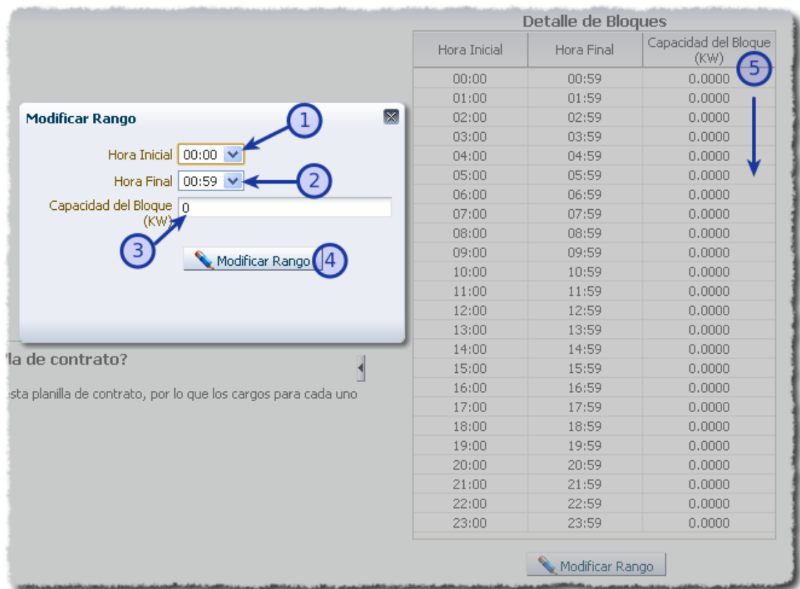
Imagen 16: Ventana de modificación de rangos de la tabla de detalle de bloques de una planilla tipo E contrato existente EEGSA-PQP bloque A y B.
