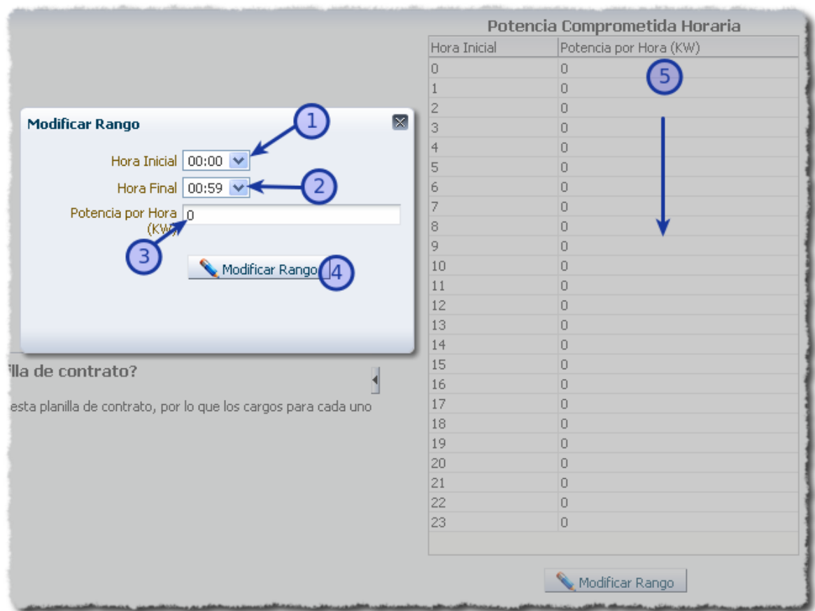
Imagen 44: Ventana de modificación de potencia comprometida por hora, planilla tipo E contrato existente EEGSA–PQP bloque C.
