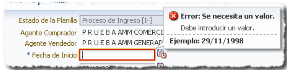
Imagen 53: Restricción de valor requerido de fecha de inicio de planilla
