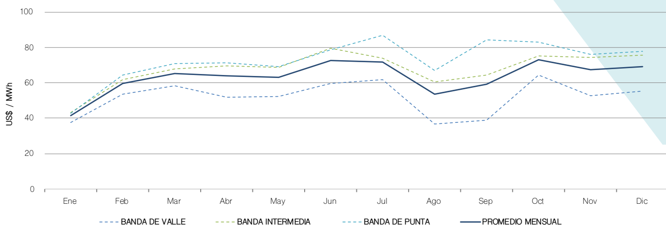
Precio promedio mensual y por Banda Horaria en el Mercado Eléctrico Regional (US$ / MWh)*
