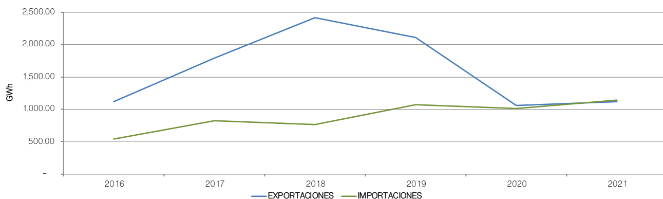
Importaciones y Exportaciones
